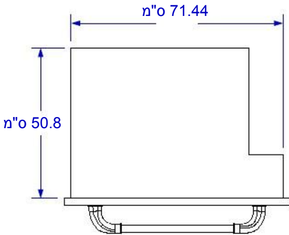
מבט עילי
