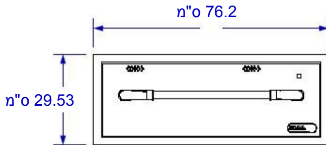
מבט חזיתי
